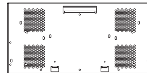
LDS32U(S)
