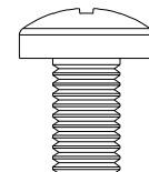
M8 x 16 mm (6) 520-9257
