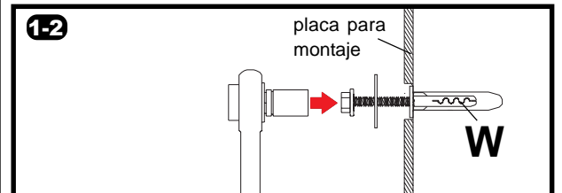
Coloque la placa sobre los anclajes y fjela con los tornillos
