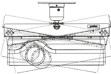
30° (±15°) ROLL
